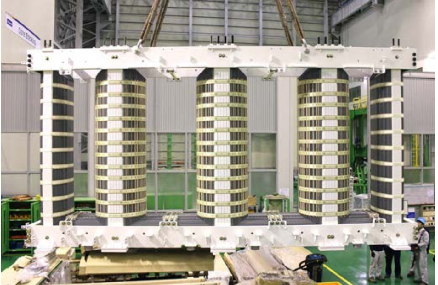
· 철심 조립
